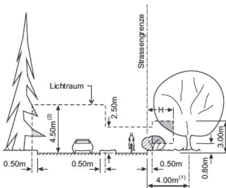
(Abbildung 1b – Lichtraumprofil mit Rad-/Gehweg)
