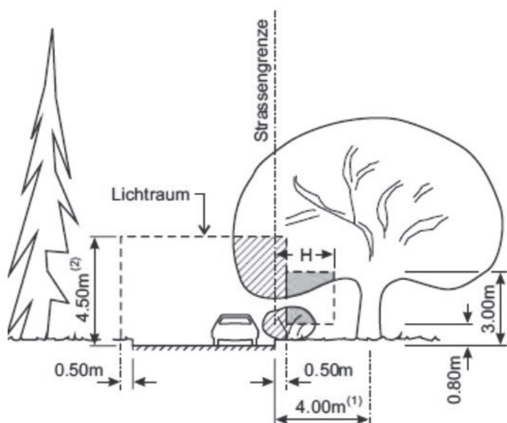
(Abbildung 1a – Lichtraumprofil)
